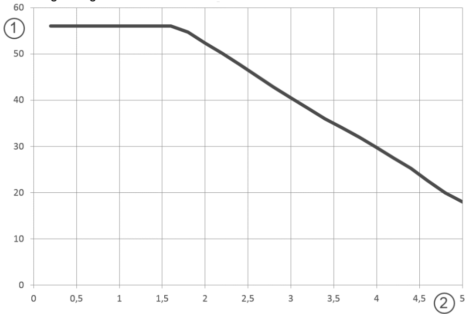
Druckerhöhungsanlage FU-X 2/40 N/NE
