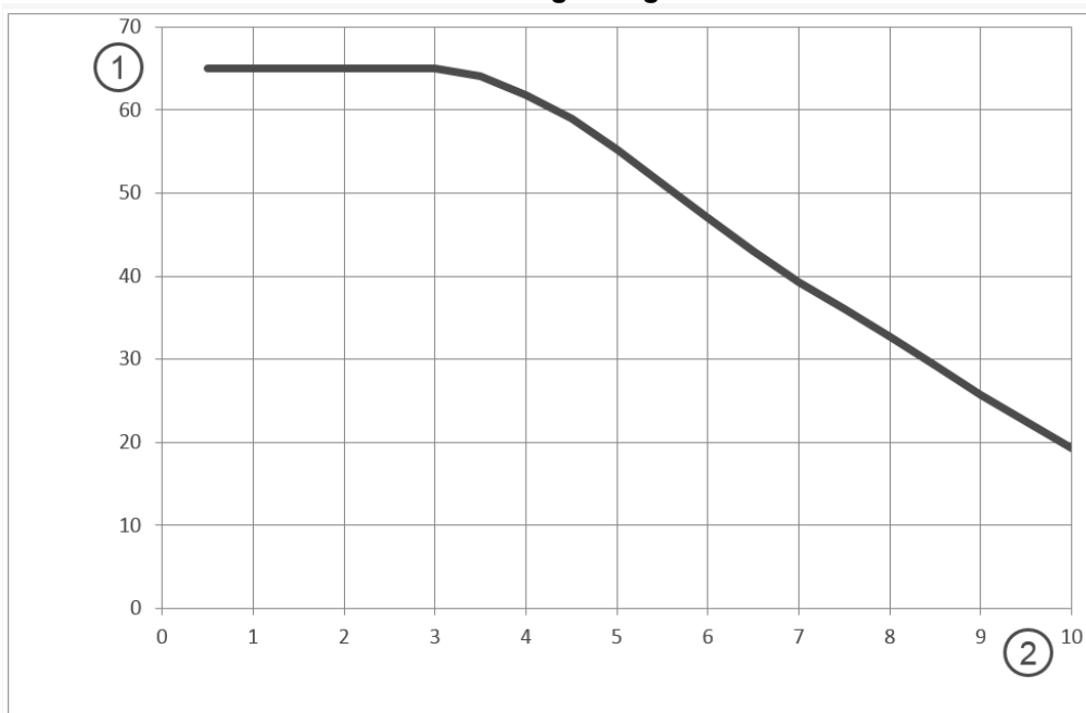
Druckerhöhungsanlage FU-X 4/40 N/NE
