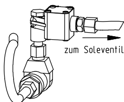
Desinfektionseinrichtung (vormontiert)
