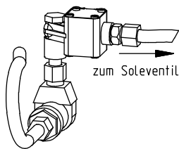
Abb. C-4 Desinfektionseinrichtung (vormontiert)
